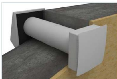
Montāža standarta sienā
